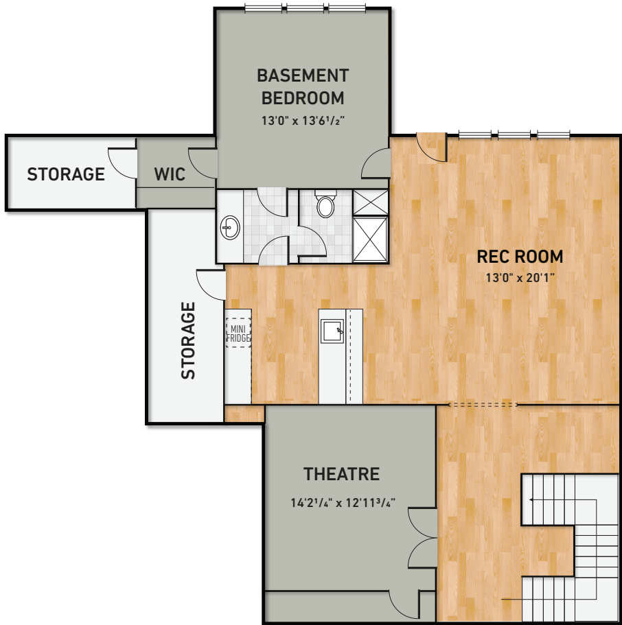
OPTIONAL BASEMENT
